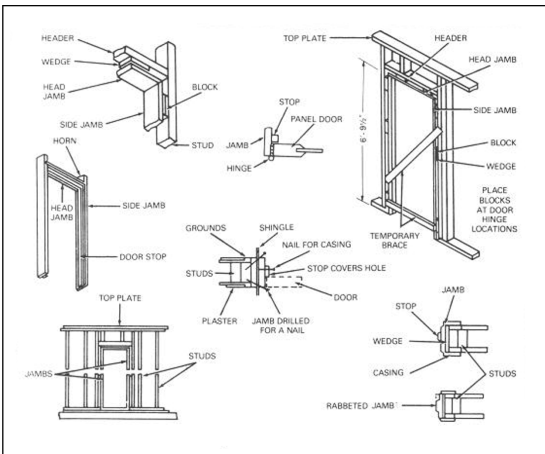
Figure 8-7. Door jambs
